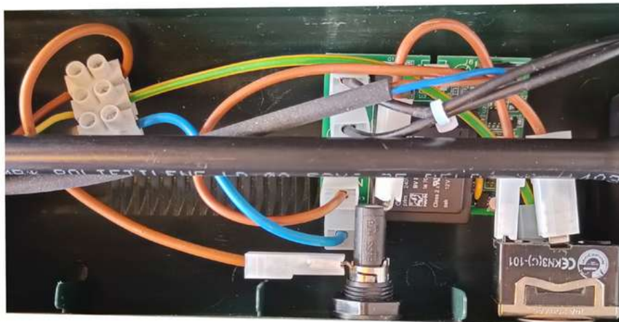
Figura 6 - Zona "Q": circuito elettrico della centralina
